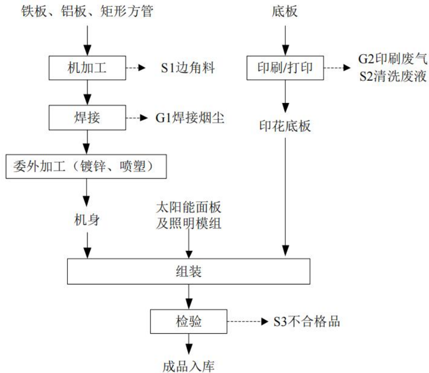
图2.3-1 本项目太阳能智能照明灯塔工艺流程及产污节点图
